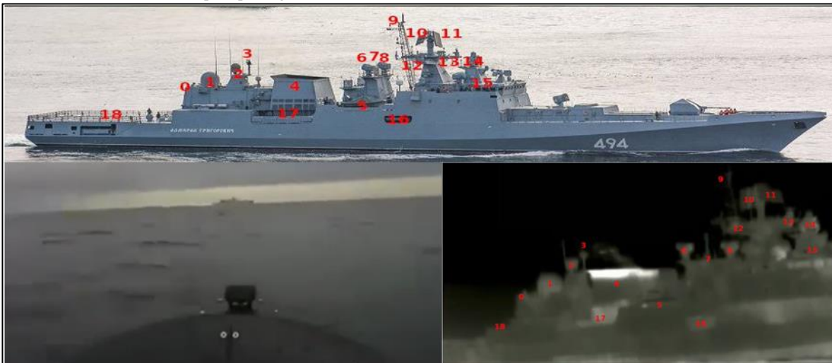
Figura 6. USV atacando a la fragata rusa Almirante Makarov el 29 de oct del 2022 y análisis de imagen térmica sobre silueta de referencia de un buque tipo fragata de la Clase Almirante Gorshkov
